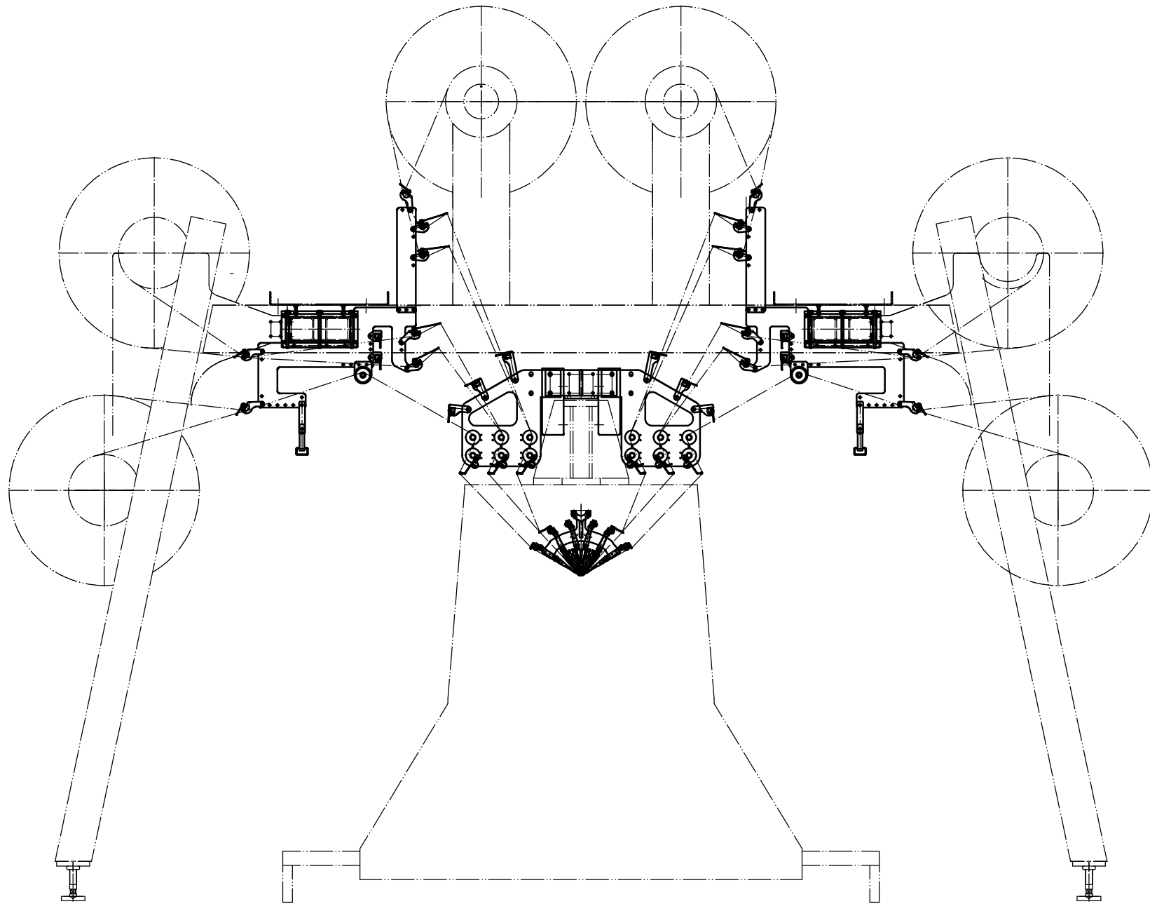
GE296DJ4-2纱路图
